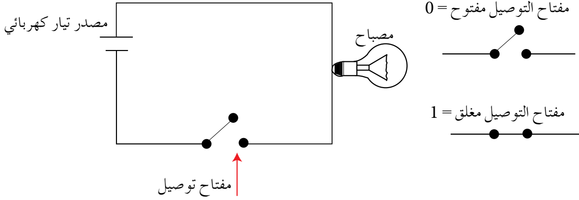
الشكل (١-٣): دائرة كهربائية بسيطة.
