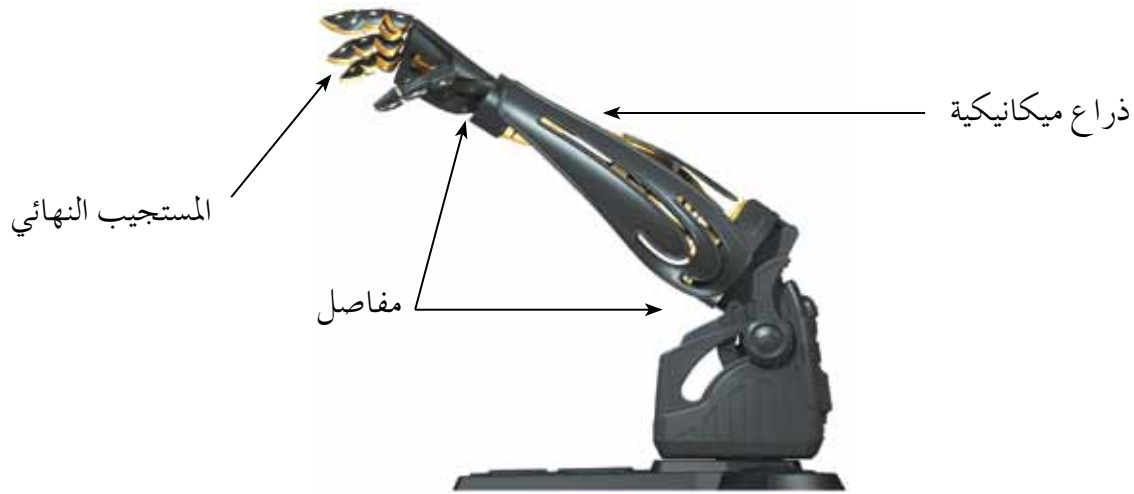
الشكل (٣-٢): مكوّنات الروبوت البسيط.
