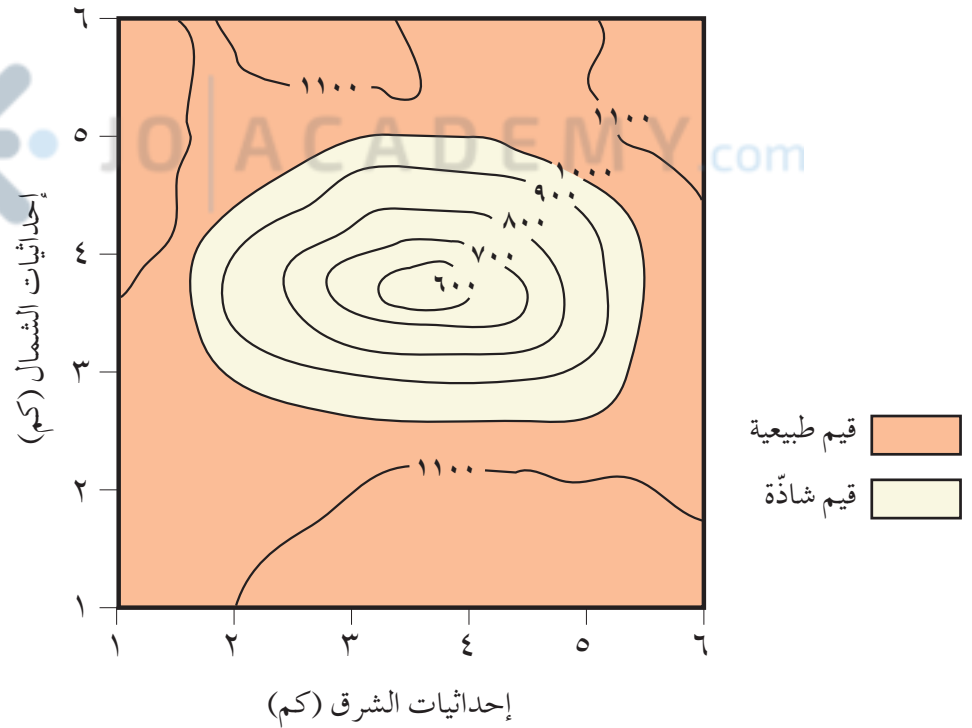
الشكل (٥-٤): خريطة كنتورية تُبيّن شاذة كهربائية سالبة، وتُقاس بوحدّة (أوم. متر).
