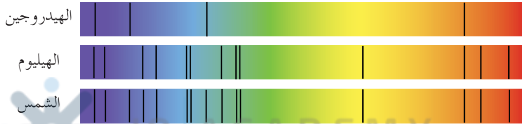
الشكل (٦-١): طيف امتصاص الهيدروجين والهيليوم في طيف الشمس. وقد تم التركيز على طيفي امتصاص الهيدروجين والهيليوم؛ لأنهما يشكّلان المكوّنات الرئيسة للشمس ونسبة ٩٨٪ تقريباً.
