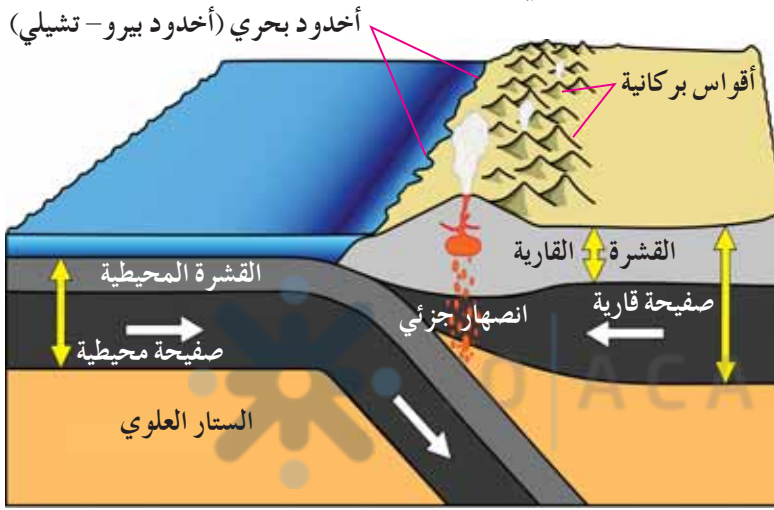
(أ) حدود غوص من نوع (محيطي - قاري).
