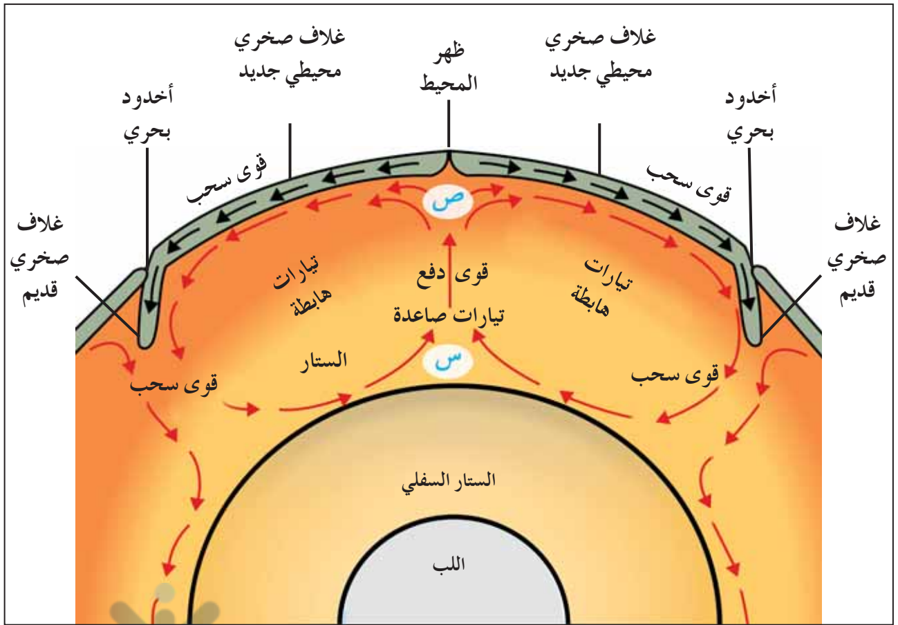
الشكل (٥-٢٠): نموذج يُفسّر القوى المحركة للصفائح الأرضية؛ تيارات الحمل وما ينتج منها من قوى الدفع عند ظهر المحيط وقوى السحب عند الأخاديد البحرية.
