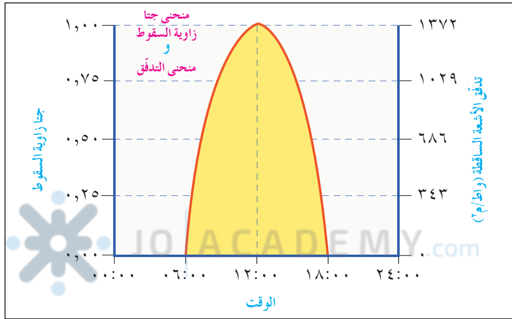
الشكل (٦-٢): تغيّر تدفق الأشعة الساقطة على السطح، بتغيّر زاوية السقوط على مدار اليوم.
