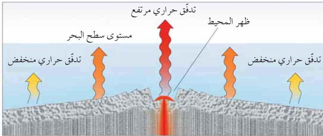
الشكل (١٣-٥): قيم التدفق الحراري عند ظھر المحيط وعلى جانبيه.
