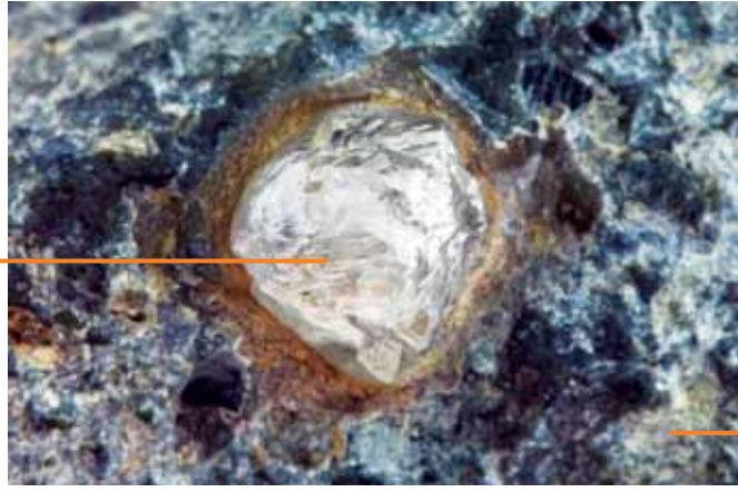
الشكل (٤-٣): صخر كمبرلايت يحتوي على قطعة من الألماس.
