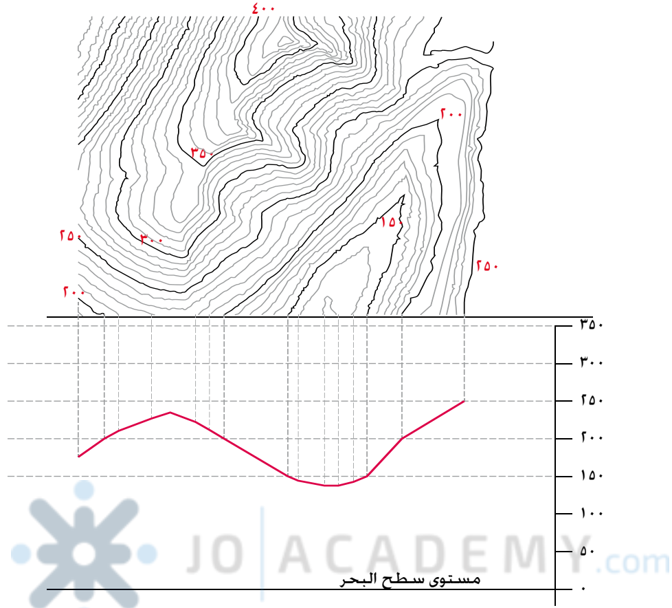
الشكل رقم (٣-٨): خطوط الكنتور الدالة على وادٍ (أ).
