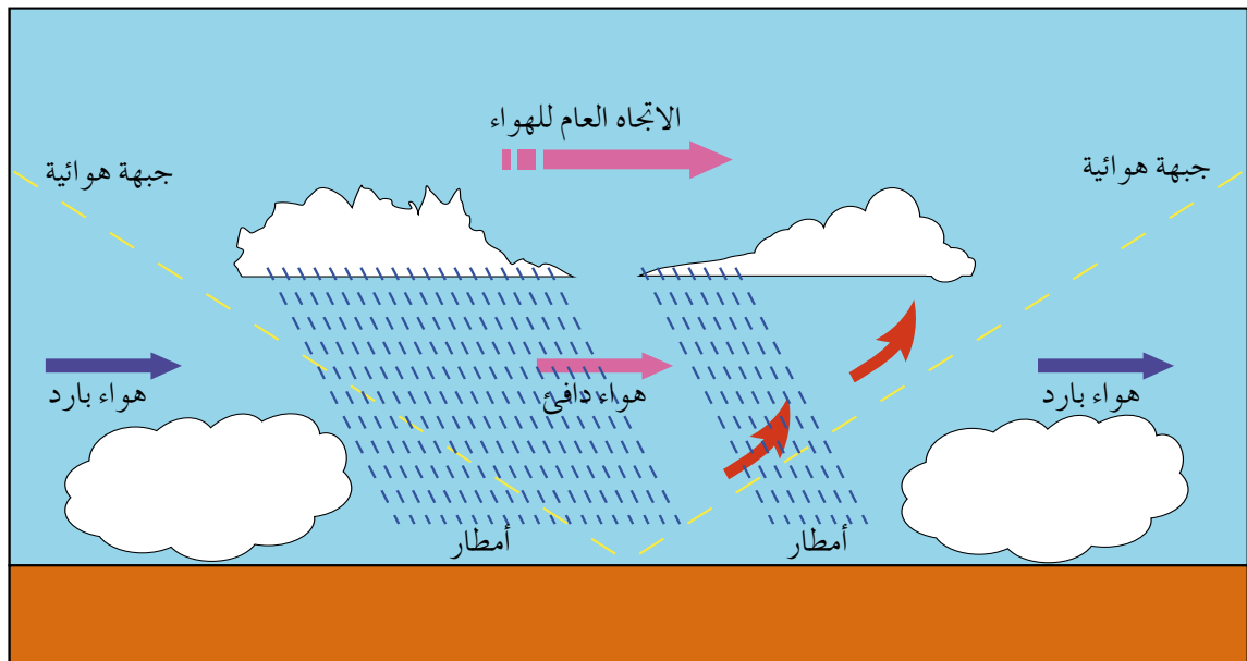
الشكل رقم (١-٩): الأمطار الإعصارية.
