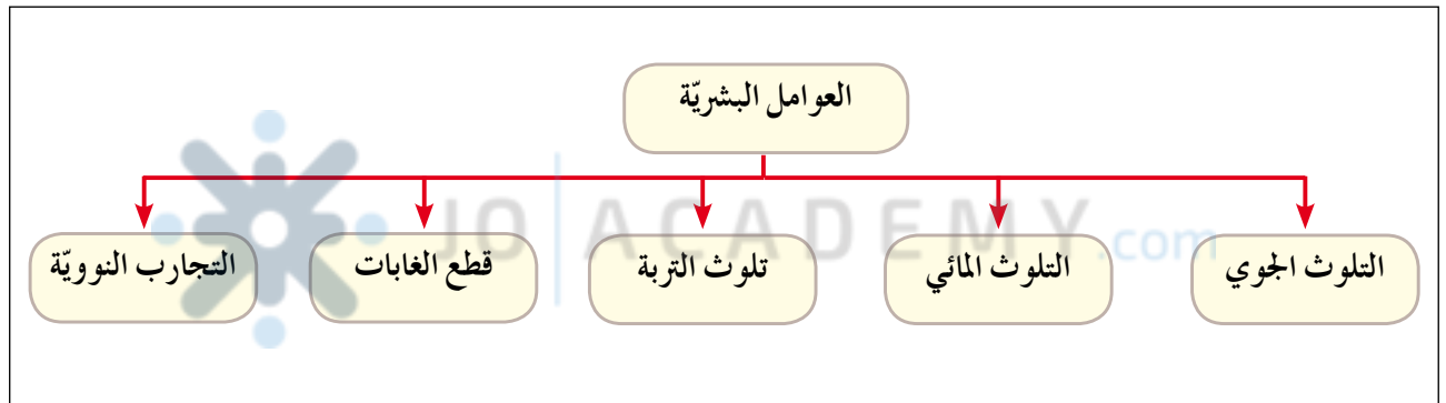
الشكل رقم (٢-٦): العوامل البشرية المؤثرة في التغير المناخي.
