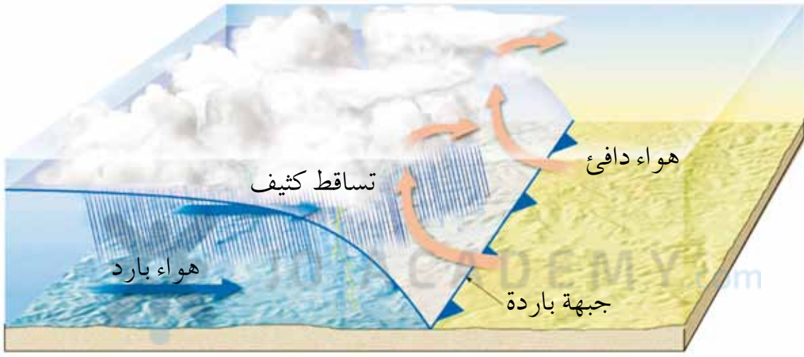
الشكل رقم (١-١٦): تكون الجبهة الهوائية.
