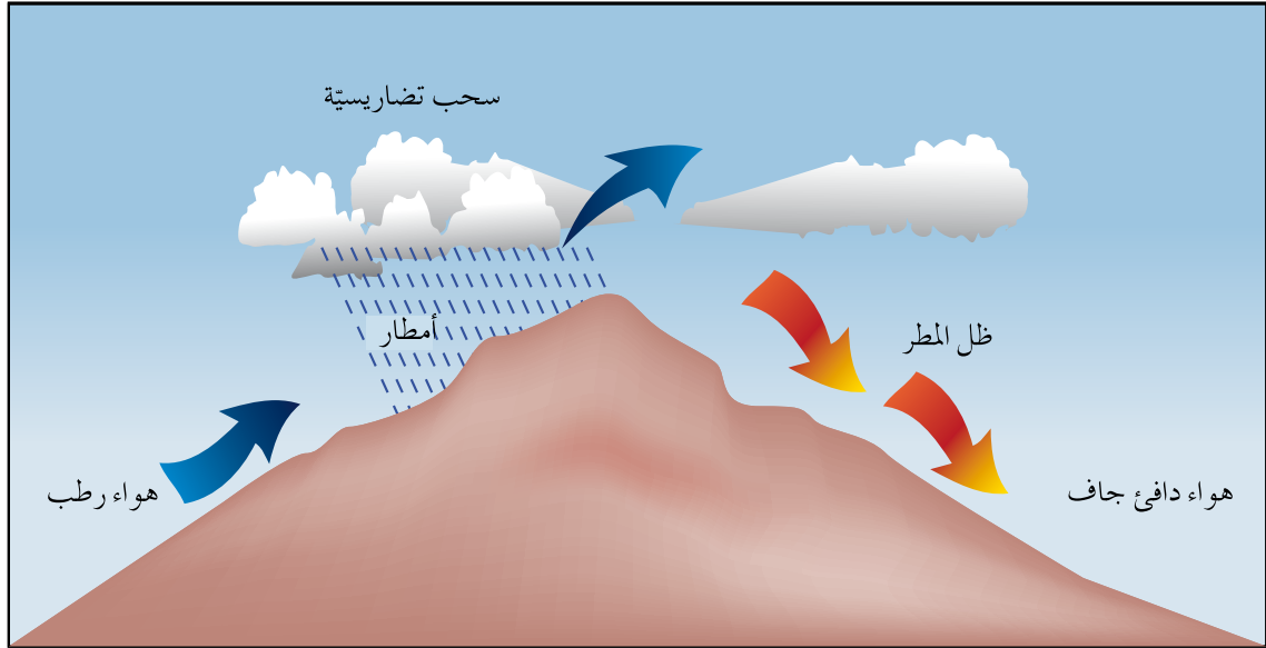
الشكل رقم (١-٨): الأمطار التضاريسية.
