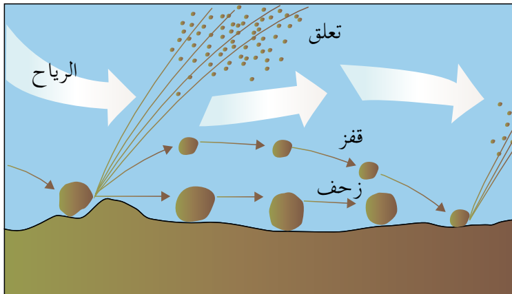
الشكل رقم (٣-١٩): طرق نقل الرياح لحواملها.
