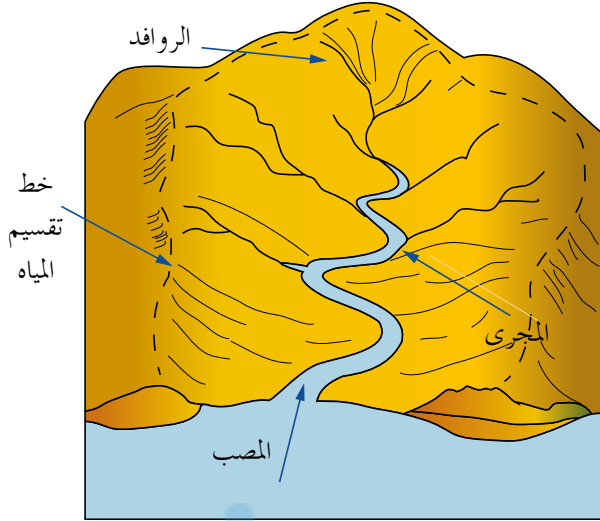
الشكل رقم (٣-٢٨): حوض نهرى.
